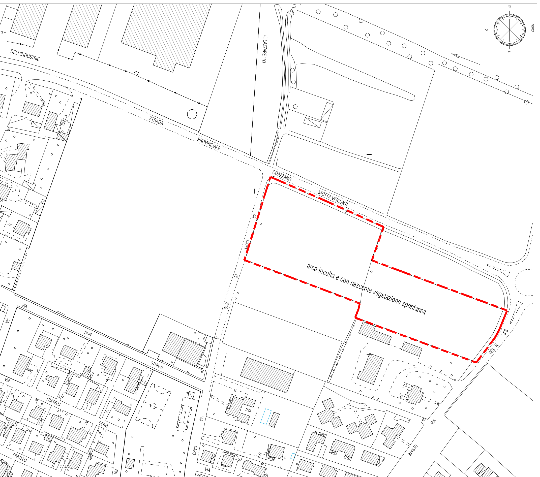
INDIVIDUAMENTO TERRITORIALE SCALA 1:5000
